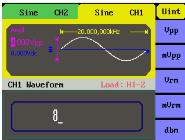
Рис. 8-3 Установка амплитуды
