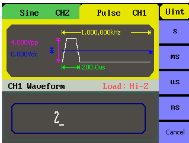
Рис. 8-10 Установка задержки
