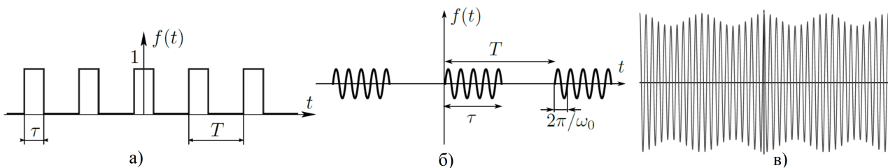
Рис. 1: Примеры сигналов а) периодической последовательности прямоугольных импульсов, б) периодической последовательности цуг, в) модулированного по амплитуде сигнала из [1]
