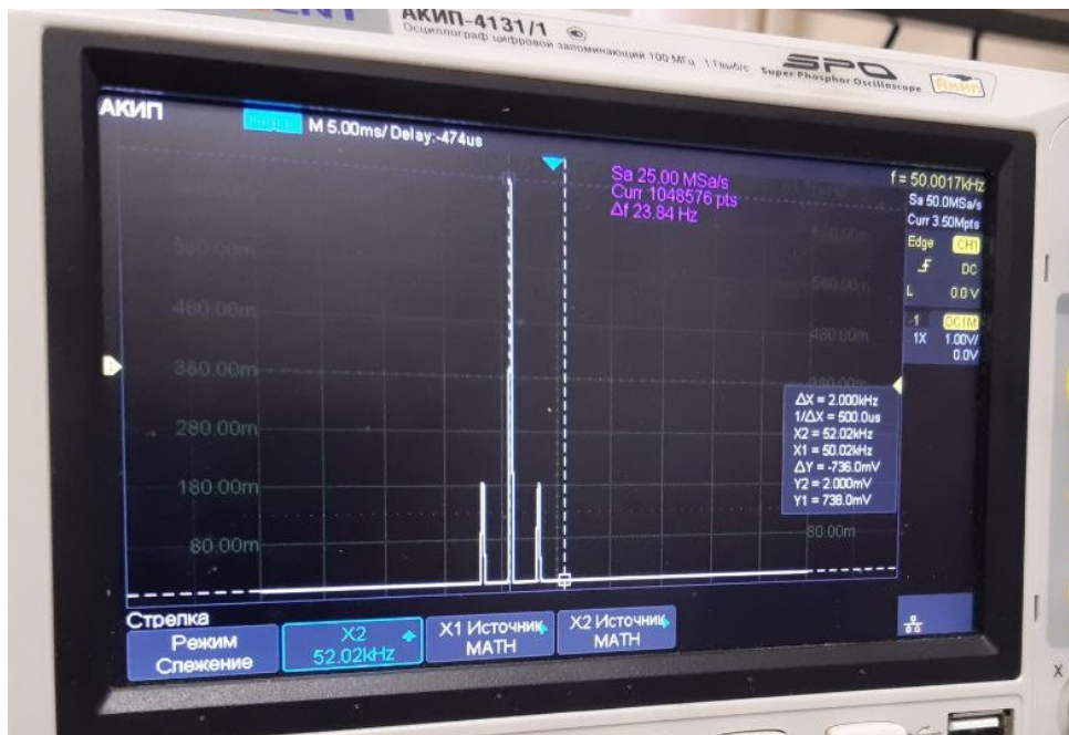
Рис. 7: Спектр сигнала, модулированного по амплитуде, при частоте несущей \nu_0 = 50 кГц, частоте модуляции \nu_{\text{мод}} = 2 кГц
