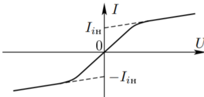
Рисунок 1.3 — Вольт-амперная характеристика двойного зонда
