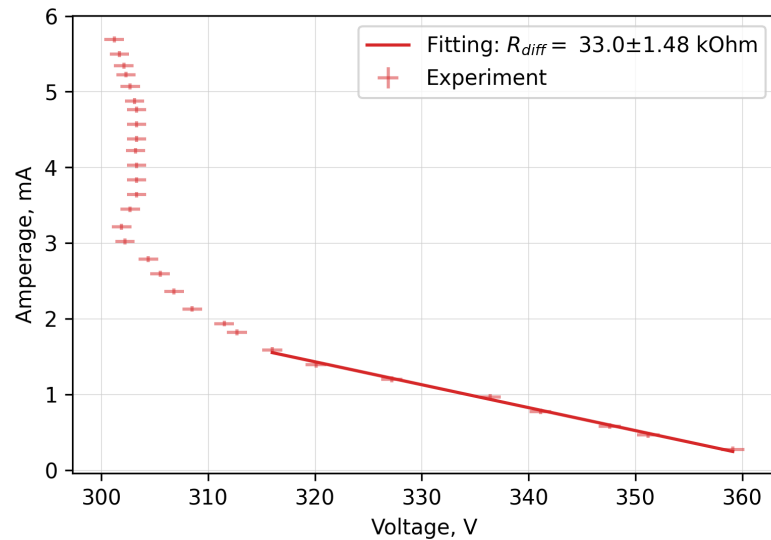
Рисунок 2.1 — ВАХ разряда
